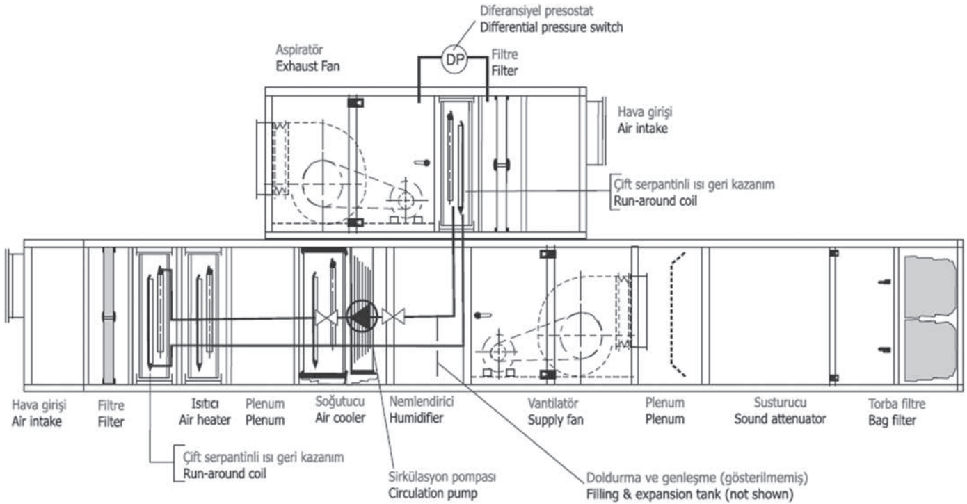
Çift Serpantinli ve Otomatik Defrostsuz Isı Geri Kazanım Sistemi. İki Katlı Santral Tazında.
