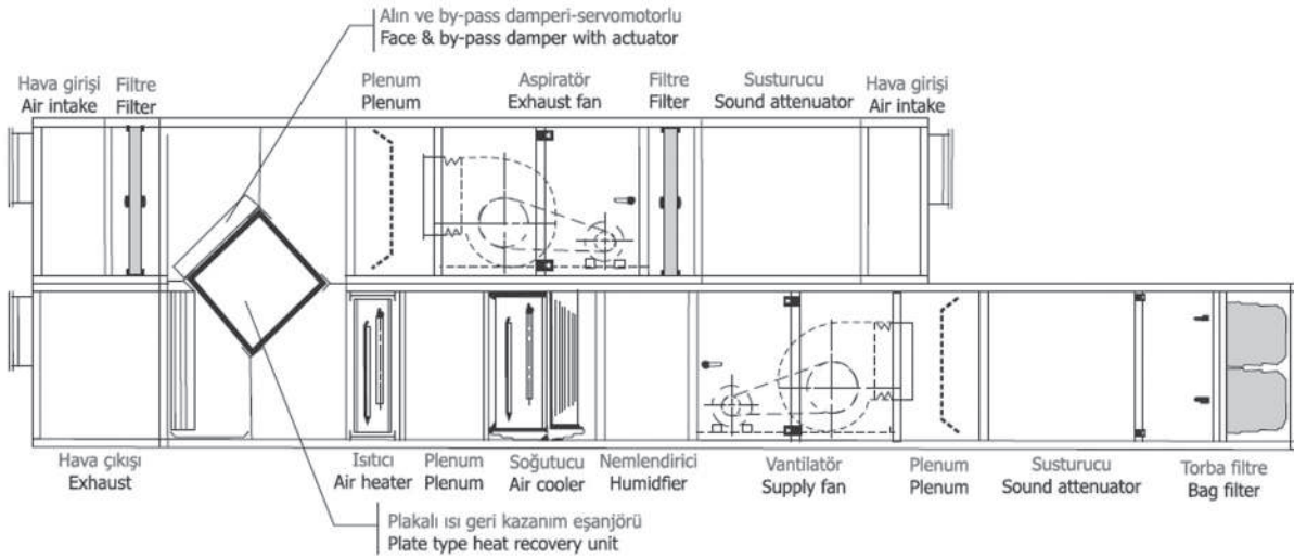
Çapraz Akışlı Isı Geri Kazanımlı Hijyenik Klima Santrali
